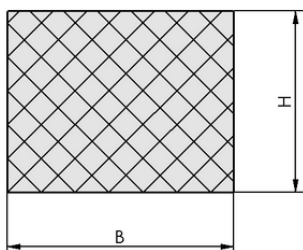
デザインデータ DI-PROF 10x6 MOS EPDM-20
