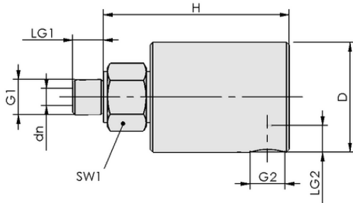
Tasarım verileri DEF R 250
