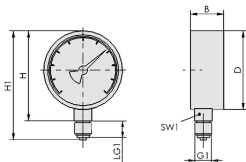
Конструктивные данные VAM 40 V U BAR
