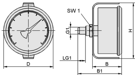
Design data VAM 67 V H-SE BAR/PSI
