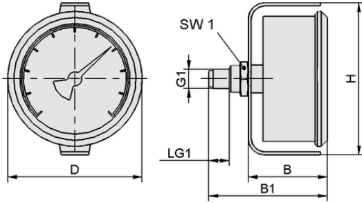
Tasarım verileri VAM 67 V H-SE BAR/PSI
