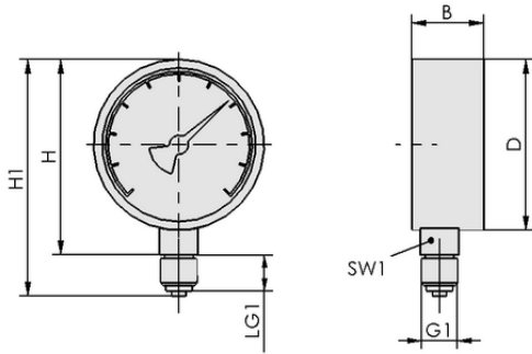
Tasarım verileri VAM 100 V250 U BAR
