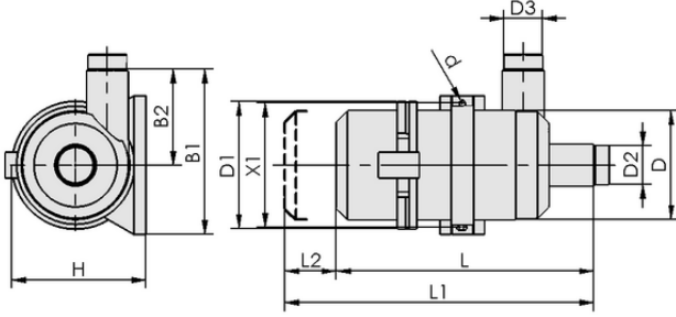
Tasarım verileri STF 110 P 12.0 SSB
