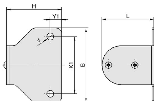
Données de construction HTR-FIL 2S WI VFT1/8-1/2
