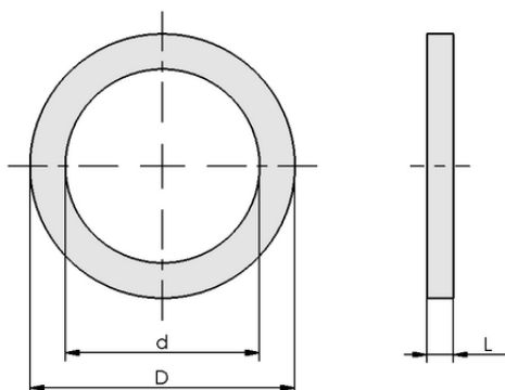
Données de construction DR 57-51x3.2 NBR
