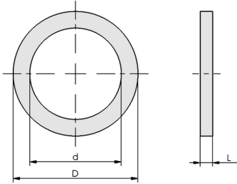
Tasarım verileri DR 37-33x3 NBR
