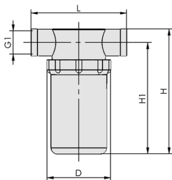
Dati di costruzione VFT G3/8-IG 100
