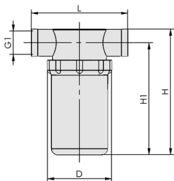
Dati di costruzione VFT G1/4-IG 80
