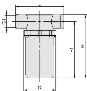
デザインデータ VFT G1/8-IG 100
