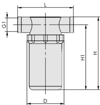
Données de construction VFT G1/8-IG 80
