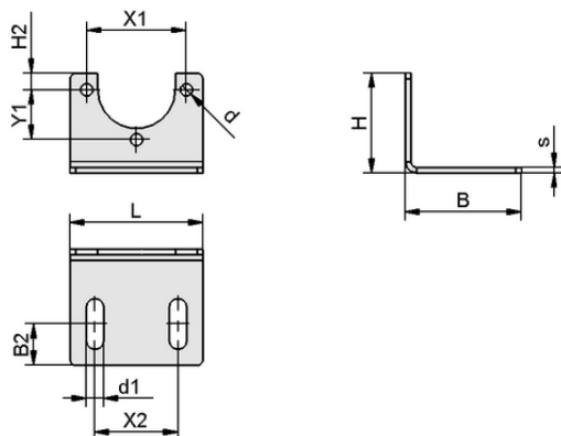
デザインデータ BEF-WIN 42x36x48 2 PVT-PVS
