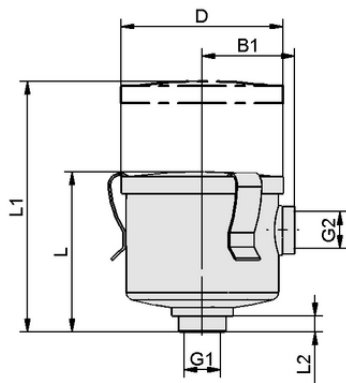
Données de construction STF G3/4-IG N
