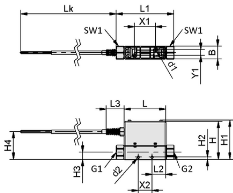
Données de construction FS 200 D 2NA K
