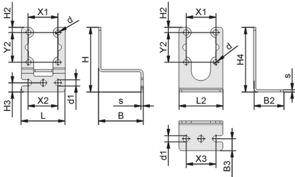
Tasarım verileri BEF-WIN 30x43.5x29.5 1.5
