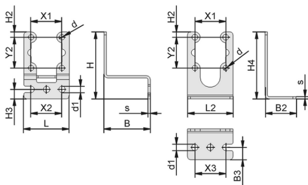
Datos de diseño BEF-WIN 20x43.5x29.5 1.5
