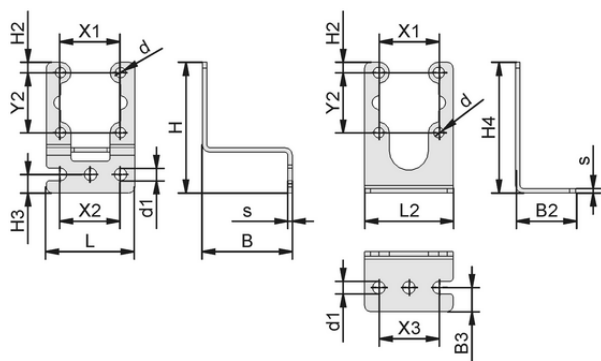
Dati di costruzione BEF-WIN 20x43.5x29.5 1.5
