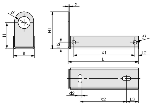
Dati di costruzione BEF-WIN 21x22x39 1.5 VSi-M8
