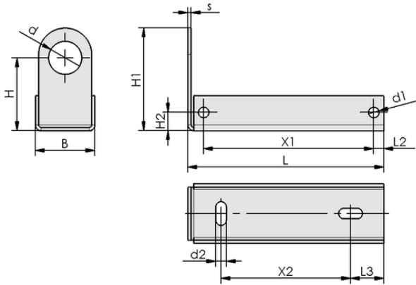
Tasarım verileri BEF-WIN 21x22x39 1.5 VSi-M8
