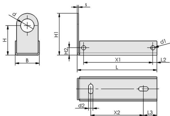
Dati di costruzione BEF-WIN 21x22x39 1.5 VSi-M12
