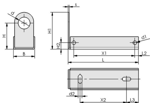
Données de construction BEF-WIN 21x22x39 1.5 VSi-M12
