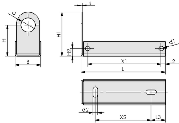
Tasarım verileri BEF-WIN 21x22x39 1.5 VSi-M12
