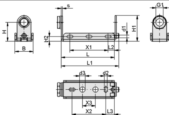
デザインデータ BEF-WIN 21x22x61.5 1.5 VSi-D-M12
