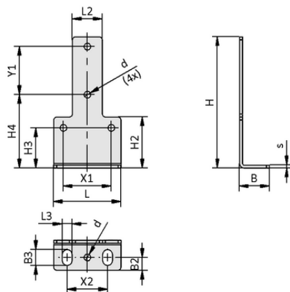
Konstruktionsdaten BEF-WIN 45x20x87.35 LQE
