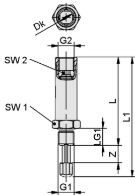
デザインデータ TV G1/8-AG 10
