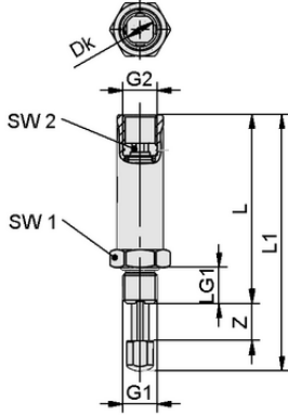
Tasarım verileri TV G1/8-AG 10
