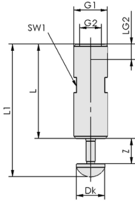
Tasarım verileri TV G1/4-AG 12
