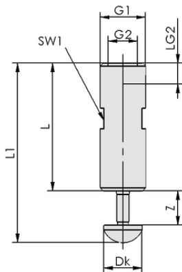
デザインデータ TV G1/4-AG 12
