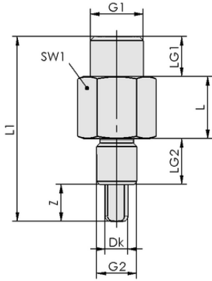
Tasarım verileri TVN G1/4-AG 9 N009
