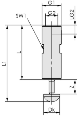
Tasarım verileri TV G1/4-AG 13
