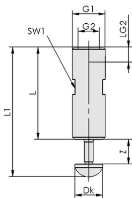
Datos de diseño TV G1/2-AG 13
