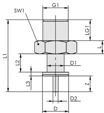
デザインデータ TVN G1/8-AG 6.5 N008
