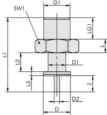
Tasarım verileri TVN G1/8-AG 6 N007
