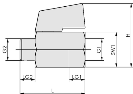
Конструктивные данные KVZ 8 2/2
