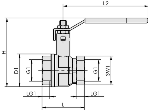
Tasarım verileri KVZ 32 2/2
