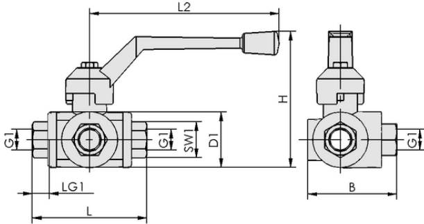
Tasarım verileri KVD 20 3/2
