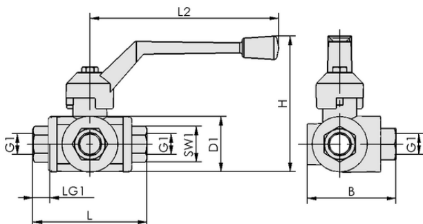
Dati di costruzione KVD 15 3/2
