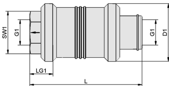
Datos de diseño HSV 12 3/2 G1/2-IG
