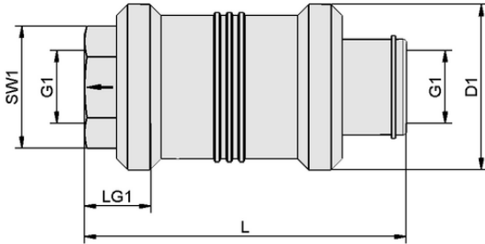
Tasarım verileri HSV 8 3/2 G3/8-IG
