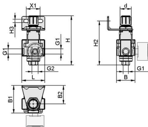
Datos de diseño VR G1/4-IG HW
