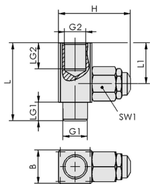
Datos de diseño DBV-M G1/4-AG MS
