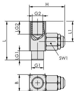
デザインデータ DBV-M G1/4-AG MS
