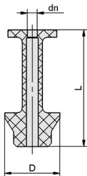
デザインデータ SW 150 P 7.3
