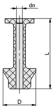
Données de construction SW 130 P 7.3
