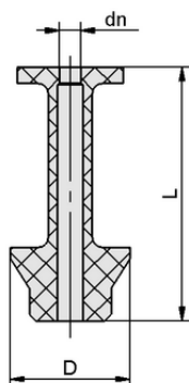
Dati di costruzione SW 100 P 7.3
