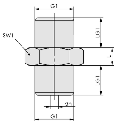
Datos de diseño SW 200 G1/4-AG
