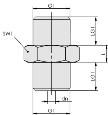
Dati di costruzione SW 120 G1/4-AG
